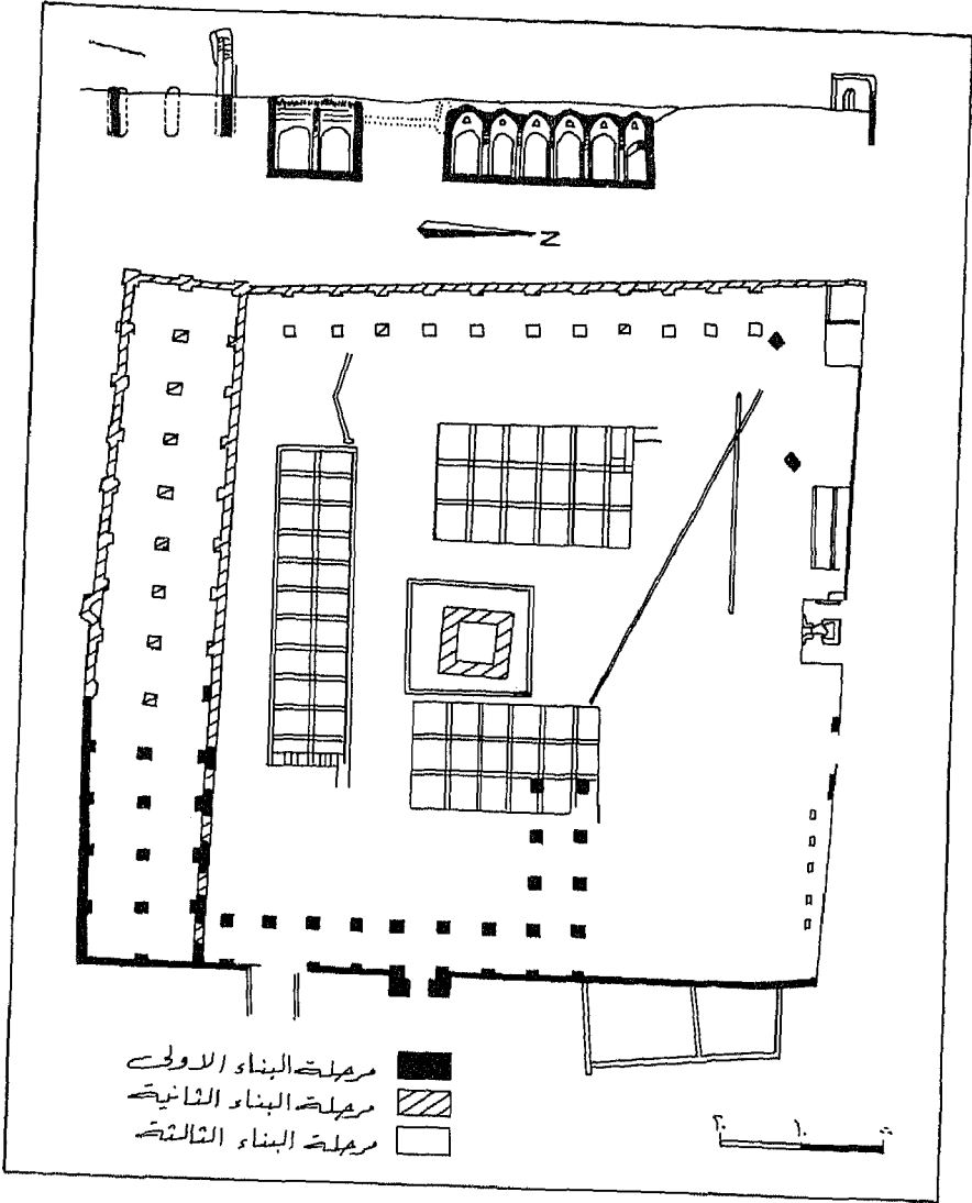
مخطط الجامع الأبيض في الرملة
