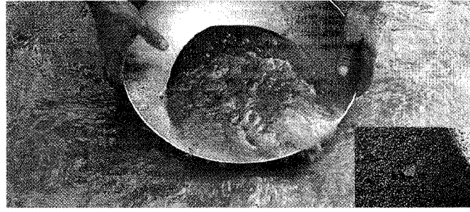
البحث عن الذهب من خلال الرسوبيات القاررة - الترسبات المعدنية - الموجودة في مجاري السيول والأنهار
