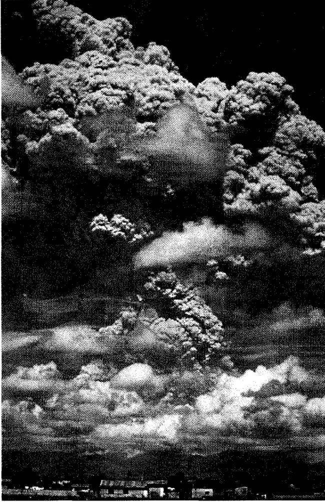
بخار يتصاعد من فوهة بركان
