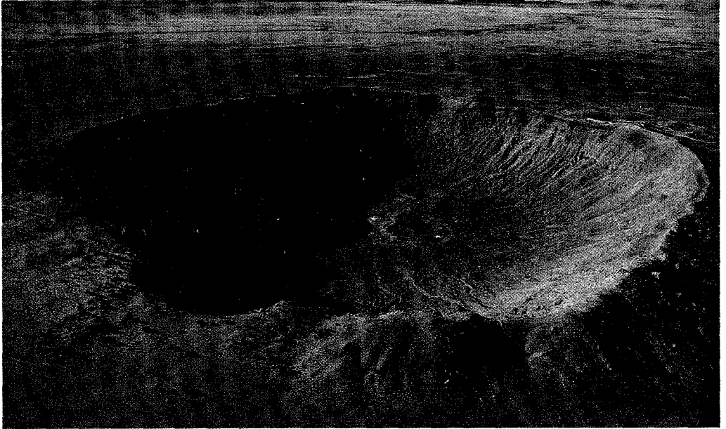
فجوة ضخمة (يبلغ طول قطرها 32 كلم تقريباً) تكونت من جراء ارتطام نيزك بأرض ولاية أريزونا
