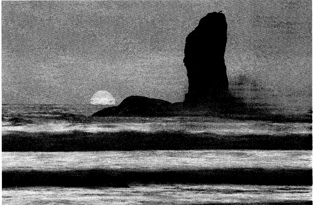
الثلوج والبحار صورة من صور توزيع الماء على سطح الأرض
