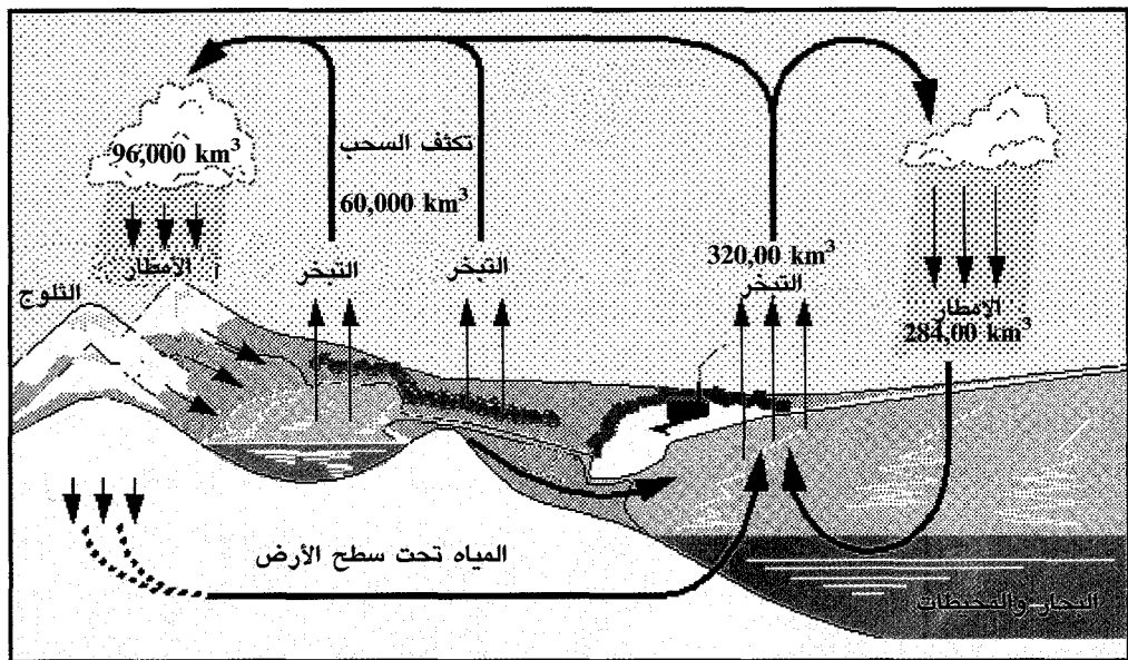
رسم تخطيطي لدورة الماء حول الأرض
